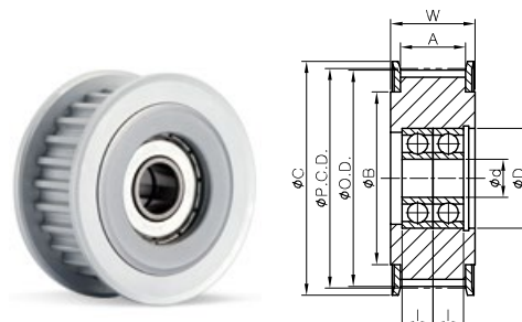
IDTCタイプ (ダブルベアリング)
