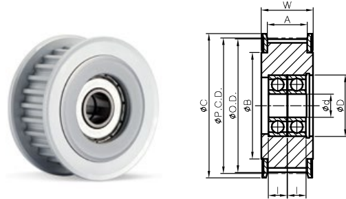
IDTCタイプ (ダブルベアリング)
