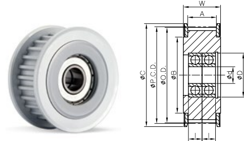
IDTCタイプ (ダブルベアリング)
