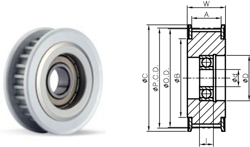
IDOCタイプ (シングルベアリング)
