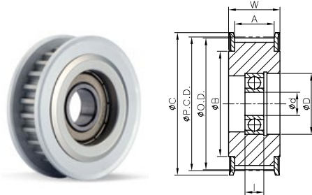
IDOCタイプ (シングルベアリング)
